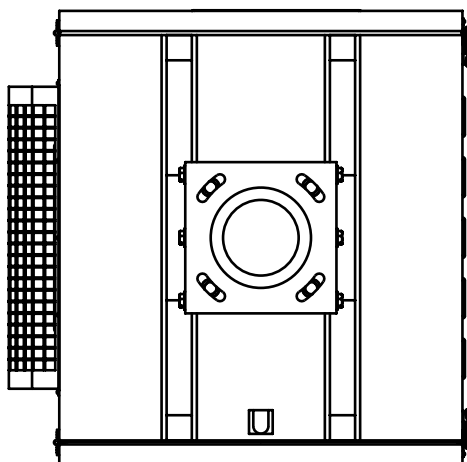
Front@1
