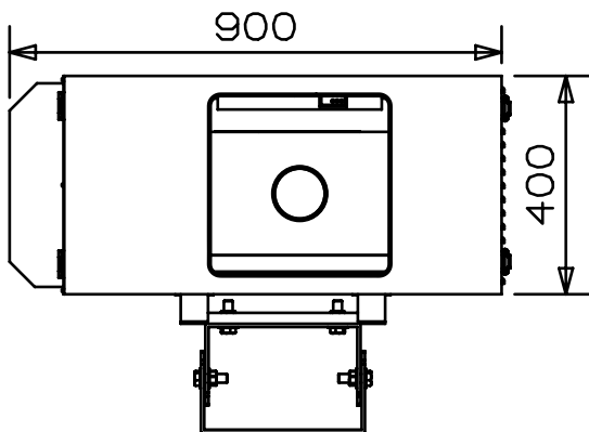
ORTHO@2
