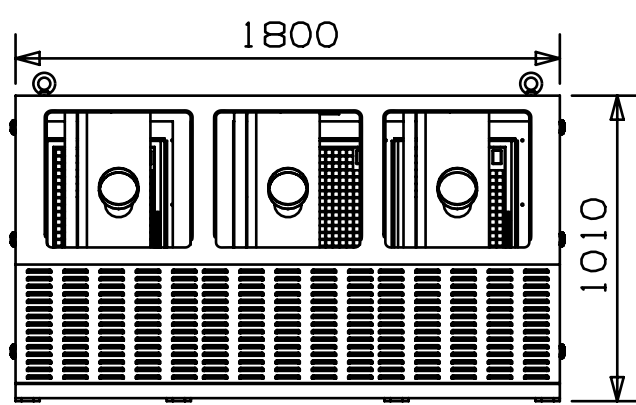
Front@1
